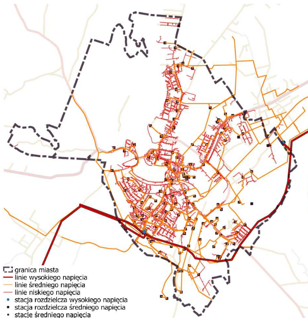
Ryc. 6. Schemat systemu elektroenergetycznego na terenie miasta Iława
