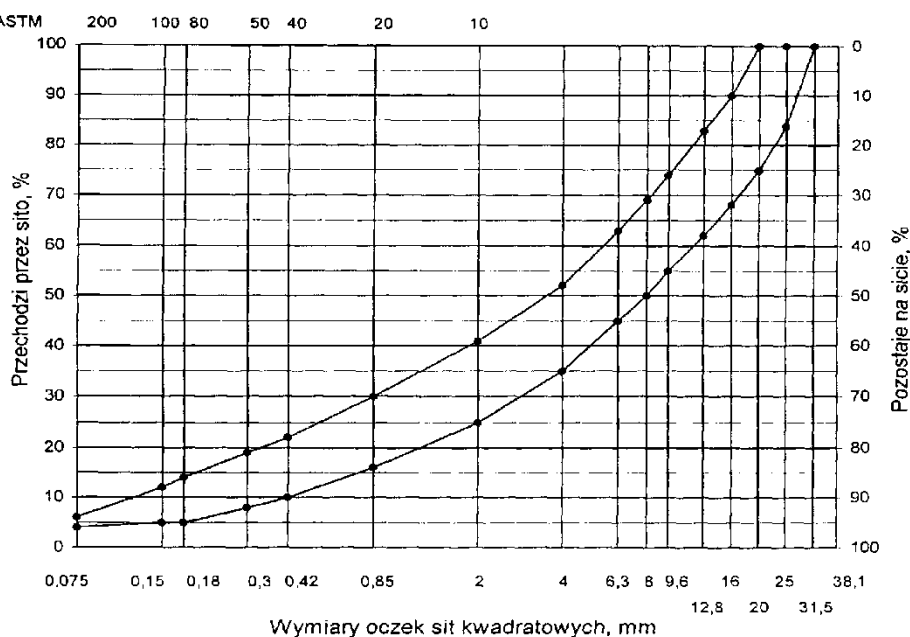
Rys. 12. Krzywe graniczne uziarnienia mieszanki mineralnej BA od 0 do 20 mm do warstwy wiążącej, wyrównawczej i wzmacniającej nawierzchni drogi o obciążeniu ruchem KR3
