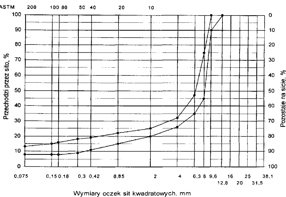
Rys. 6. Krzywe graniczne uziarnienia mieszanki mineralnej SMA od 0 do 9,6 mm do warstwy ścieralnej nawierzchni drogi o obciążeniu ruchem od KR3 do KR6
