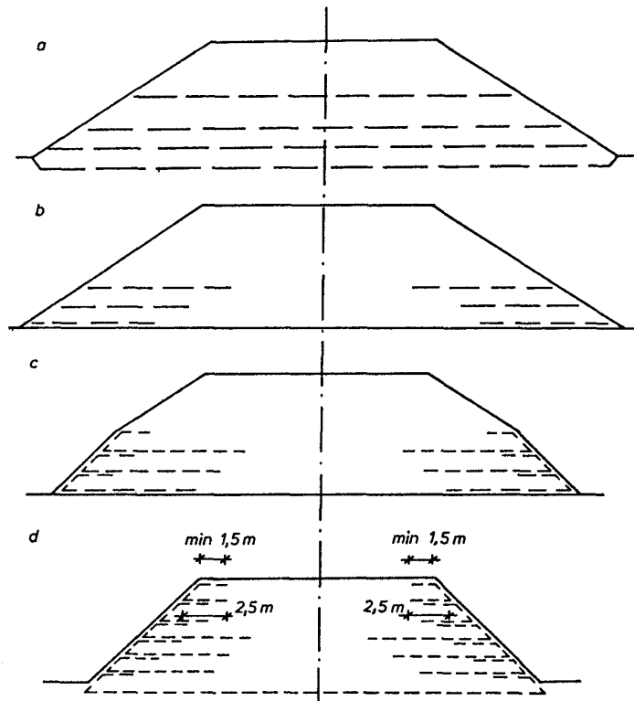
Rys. 3.2. Sposoby wzmocnienia nasypów geowłókniną
