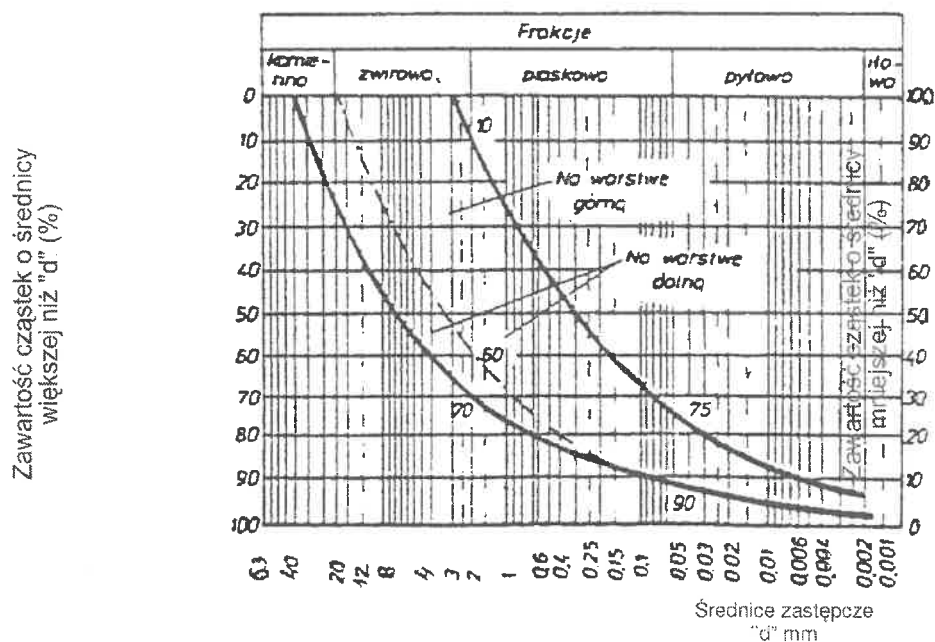
Rysunek 2. Obszar uziarnienia optymalnych mieszanek gliniasto-zwirowych
