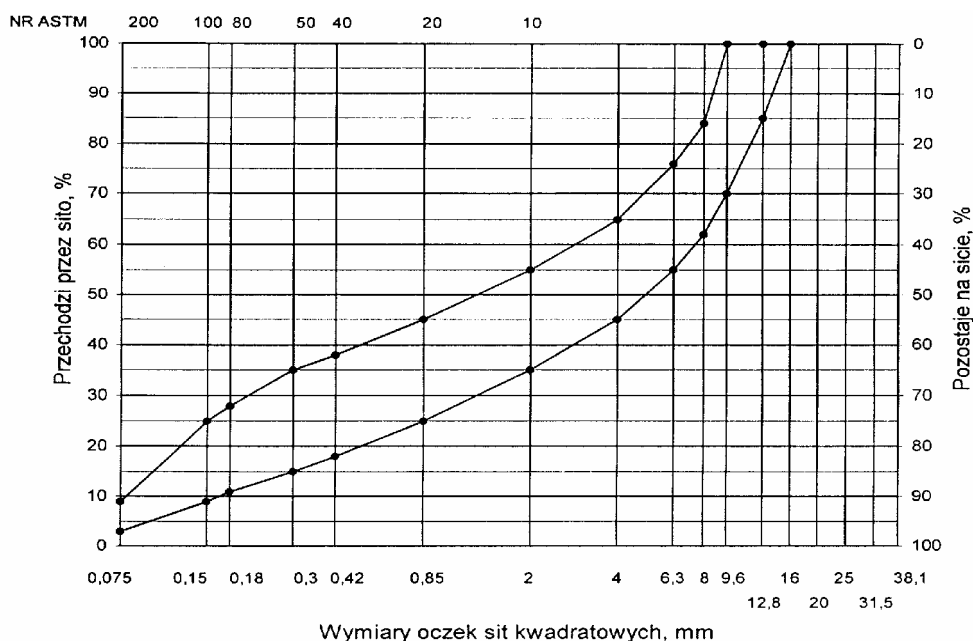
Rys. 1. Krzywe graniczne uziarnienia mieszanki mineralnej BA od 0 do 12,8 mm do warstwy wiążącej nawierzchni drogi o obciążeniu ruchem KR1 lub KR2
