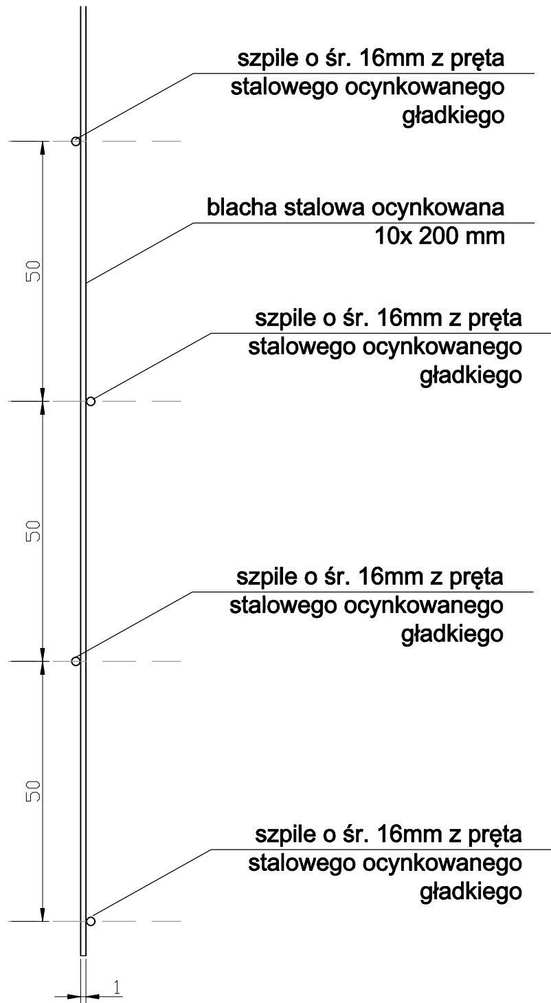
WIDOK Z GÓRY 1:10
